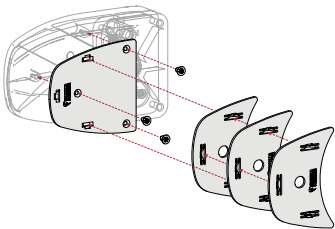
Safe Door Guardian Transit > 2006 < 2014
