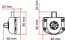
Safe Door Guardian Transit < 2006
